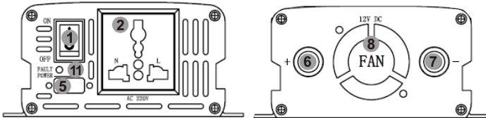
BEP300SA/BEP500SA面板示意图
