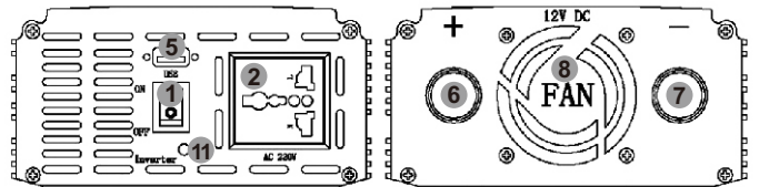
BEP1000SA面板示意图
