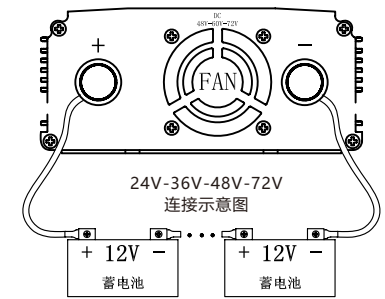
24V-36V-48V-72V连接示意图
