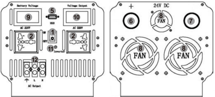
BEP5000S面板示意图
